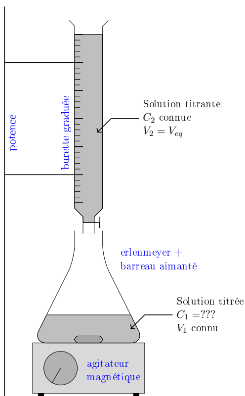
Titration colorimétrique
