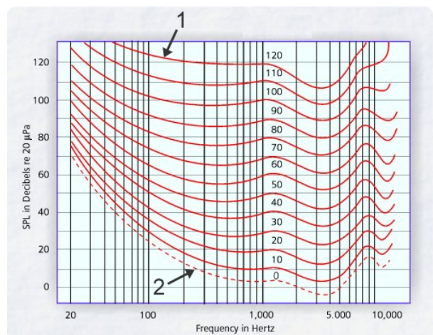
1 : seuil de la douleur, 2 : seuil d'audibilité
